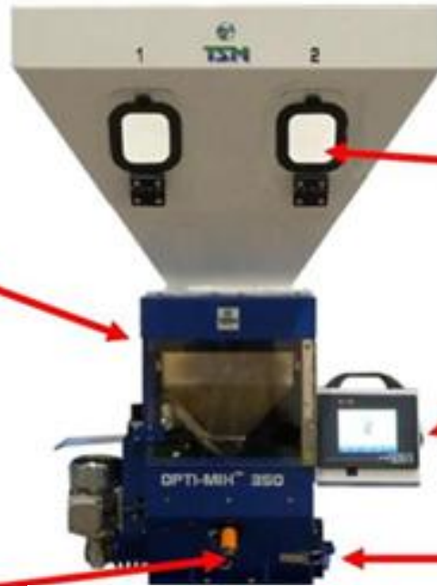
OPTI-MIX 350 CHARGEN-MISCHER
